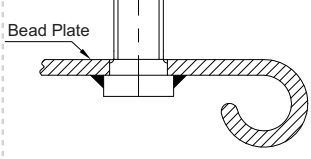
Bolt / Stud
