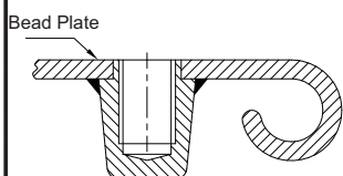
Blind Nut
